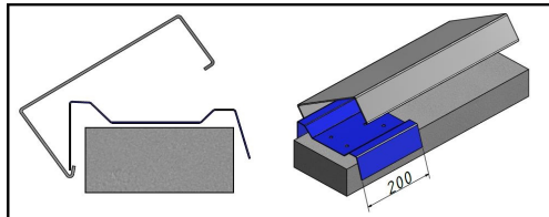
Variante 2: Halblech mit Gefälleausbildung d.h. Gefälle wird durch Halblech realisiert
