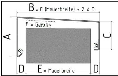
Variante 1: Standardabdeckung
