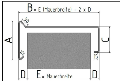
Variante 2: Mit Dreikant ohne Gefälle
