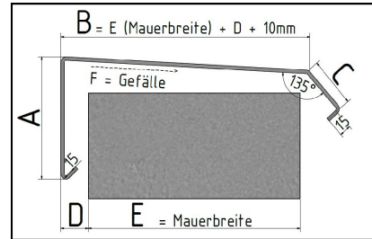
Variante 3: Dachrandabschluss
