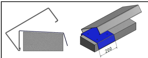
Variante 1: Halblech ohne Gefälleausbildung d.h. Gefälle wird durch Unterkonstruktion realisiert
